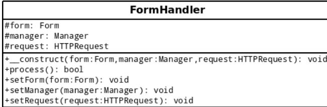
FIGURE 22.7 – Modélisation de la classe FormHandler
