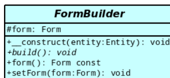
FIGURE 22.5 – Modélisation de la classe FormBuilder
