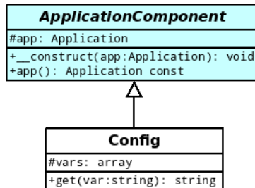
FIGURE 19.11 – Modélisation de la classe Config
