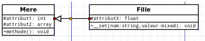
FIGURE 15.11 – Modélisation d’un héritage simple
