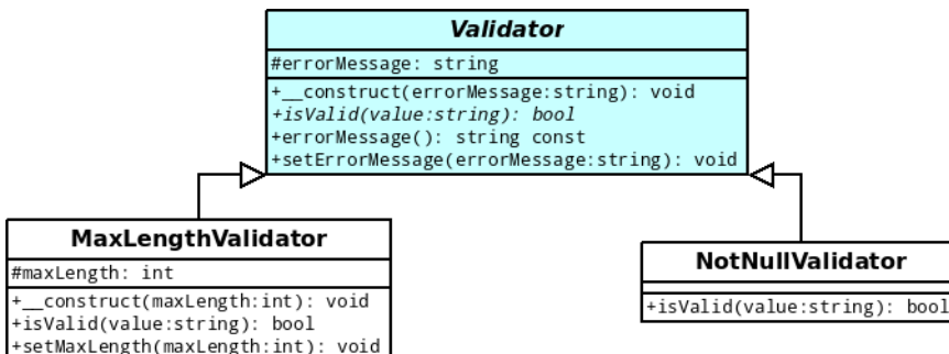
FIGURE 22.4 – Modélisation des classes MaxLengthValidator et NotNullValidator
