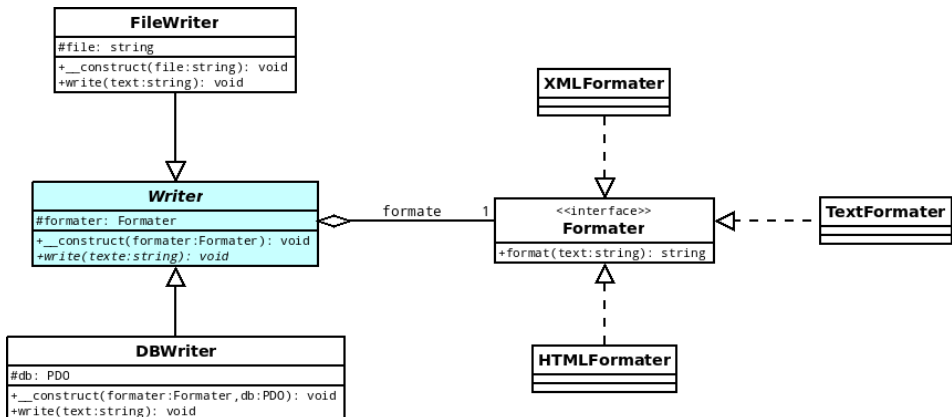
FIGURE 16.2 – Diagramme modélisant une mise en place du design pattern Strategy
