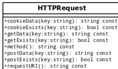
FIGURE 19.1 – Modélisation de la classe HTTPRequest
