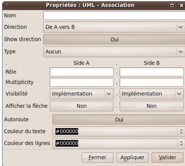
FIGURE 15.16 – Paramétrer l'association
